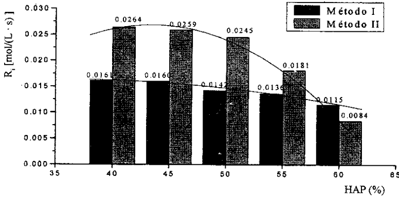
Fig. 5. Resultados correspondientes al estudio de la influencia del contenido de HAP (% p/p) sobre la velocidad inicial del proceso de fotopolimerización ( R_i ) de composites preparados por los métodos I y II, manteniendo constante el contenido de CHI (% p/p) igual a un 15 % con respecto al AA.
